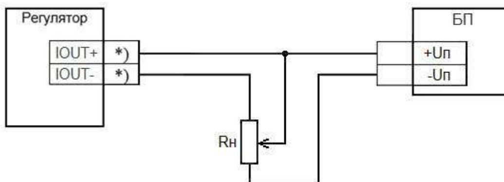
Рисунок 6. Схема подключения аналогового выхода.
